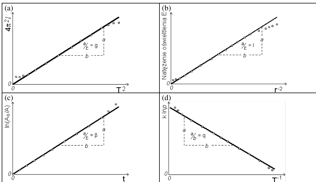
Rys. 10.2 Przykłady wyznaczania wielkości fizycznych: (a) natężenia pola grawitacyjnego g ,
