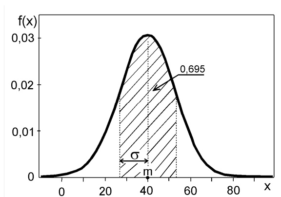
Rys. 10.1 Rozkład Gaussa.
